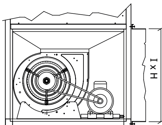
Anschluss Lufteintritt
