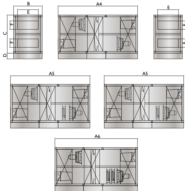
Airstream HWX mit Außenluftklappe*
