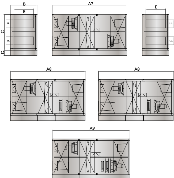
Airstream HWX mit Außenluftklappe und Rezirkulationsklappe*
