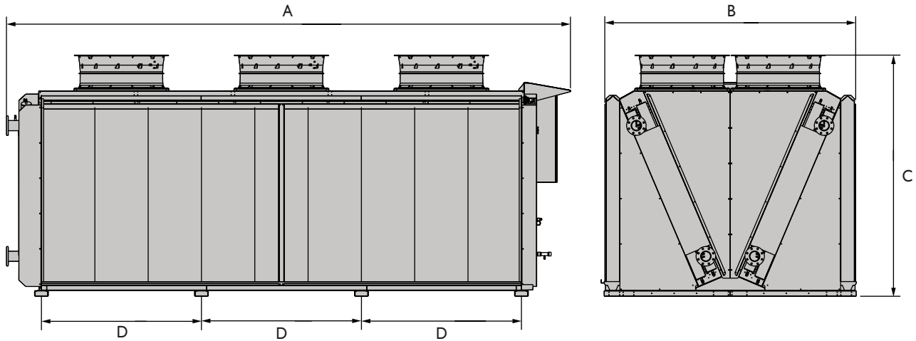
AWSD-EPA Serie – Ø 910 mm Ventilatoren – Standardversion
